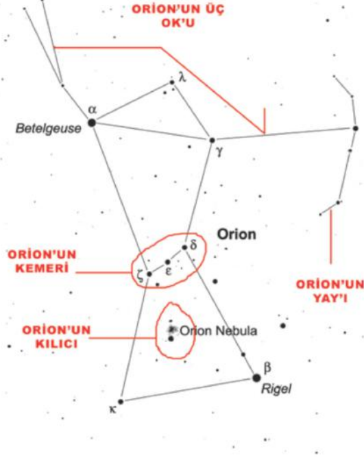
Resim 7: Orion Takımyıldızındaki üç ok ve bir yay diagram çizimi, Oğuz Kağan Destanı'nda, Oğuz'un üç ok ve bir yay'ını ifade eder. Orion'un kılıcı ve kemeri ise Oğuz Kağanı'n kemeri ve kılıcını karşılar.
