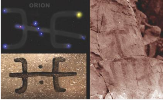
Resim 12: Afrikadaki Dogon Kabilesi'ne ait, Orion Takımyıldızı diyagramı ve Hakasya'daki Türklerin "Ediz" okunan ve Orion Takımyıldızı izdüşümü olarak çizilen tamga.
