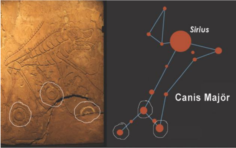
Resim 18: Canis Major köpek ya da Kurt Takımyıldızı. Takımyıldızdaki en parlak yıldız "Sirius"’tur. Yenisey’deki bu petroglif Canis Major Takımyıldızı çizimidir.
